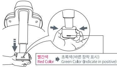
카시트 베이스 바닥 면에 수납되어 있는 서포트 레그를 앞으로 당겨 준다. Unfold the support leg out of stocking in base bottom.
