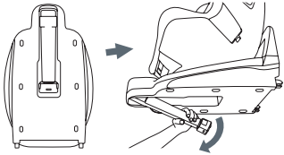
카시트 베이스 바닥 면에 수납되어 있는 서포트 레그를 앞으로 당겨 준다. Unfold the support leg out of stocking in base bottom.
